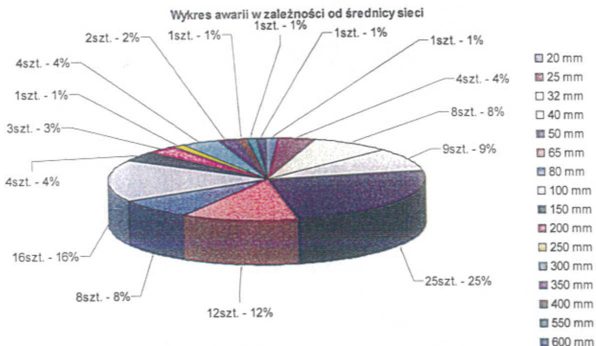
Wykres 1. Podział awarii wodociągowych w zależności od średnicy rurociągu.
